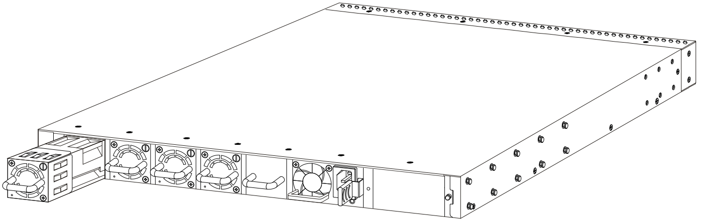
Figure 5-11 Installing Fan Module into the Fan Module Slot (Before)
